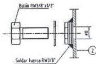
③ DETALLE TOMA DE TIERRA (TT) COLUMNA ESCALA 1:2 MATERIAL: LATÓN (Cu62-Zn36-Pb2)
