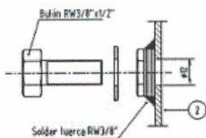
③ DETALLE TOMA DE TIERRA (TT) COLUMNA ESCALA 1:2 MATERIAL: LATON (Cu92-Zn15-Pb3)
